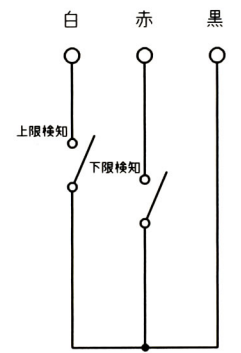
結線図
