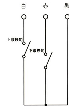
結線図
