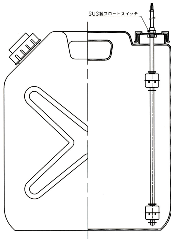
取付状態
