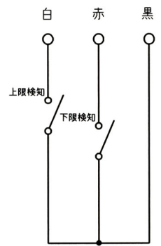
結線図
