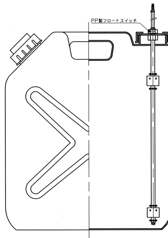
取付状態
