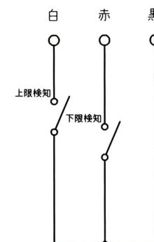
結線図
