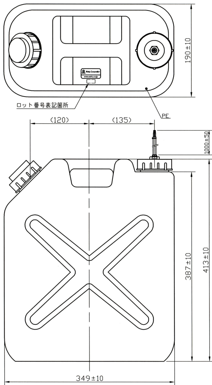
タンク寸法
