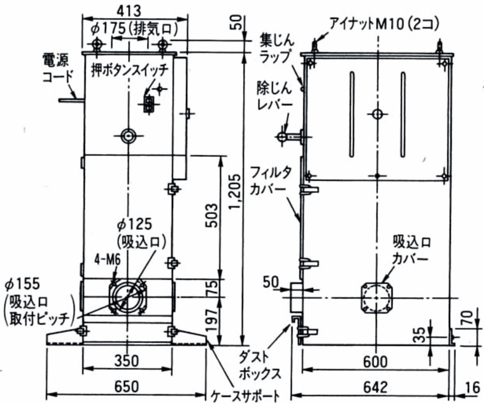
ケースサポート(標準付属品)寸法
