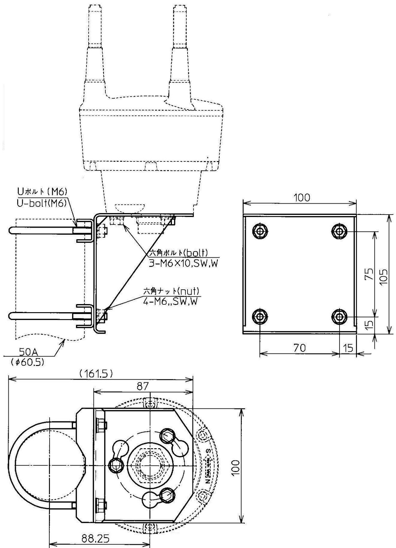
超音波風向風速計用50A取付金具 M1145S-K50A
