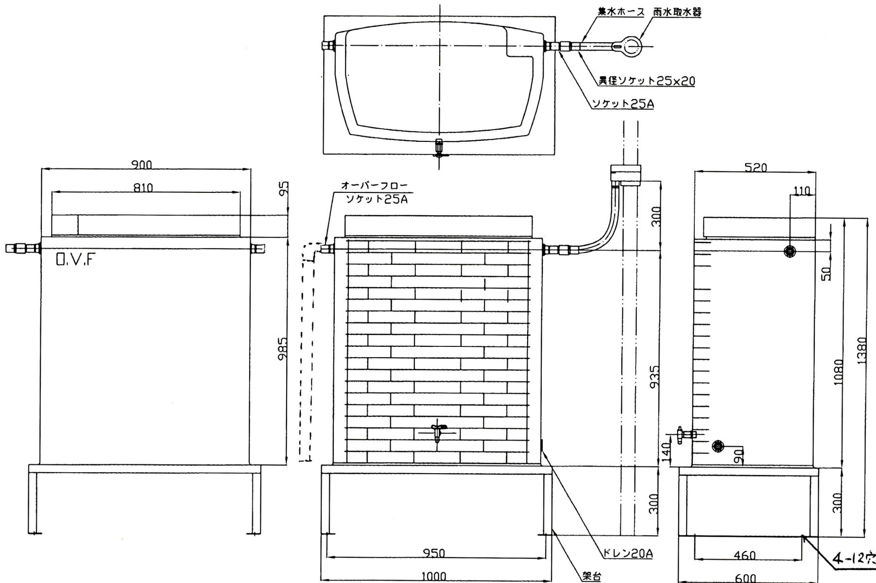
雨水タンク 尺度 M1360C2014S-200LS 1:10
