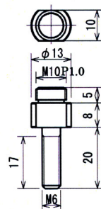
[B-8] 専用取付ボルト
