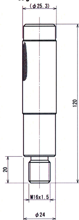
[B-7] 専用ハンドル
