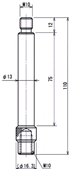
[B-6] 接続ロッド
