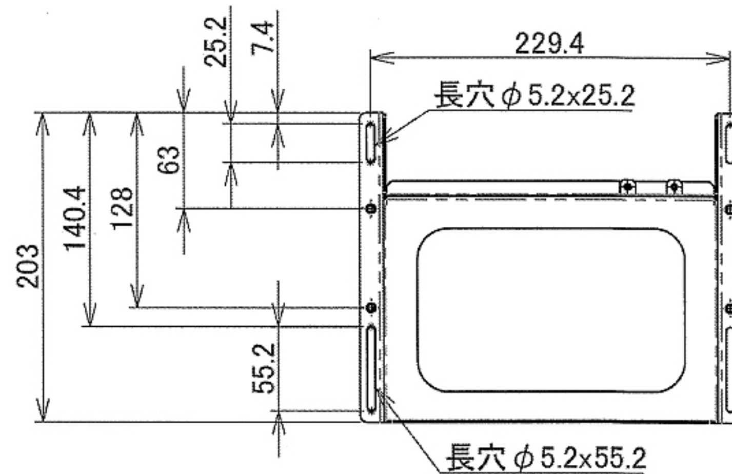
ベースブラケット取付穴寸法
