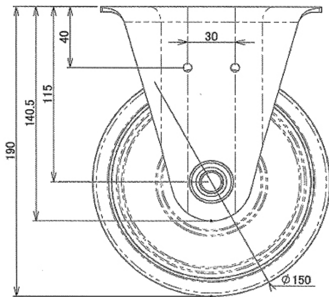
キャスター寸法
