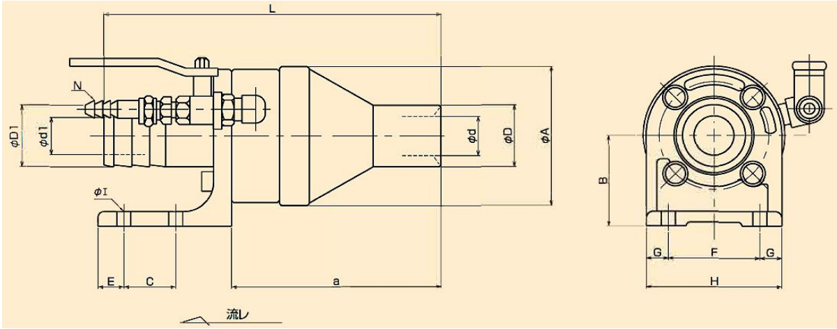
■ M472K-10B～M472K-75B寸法表（標準品）
