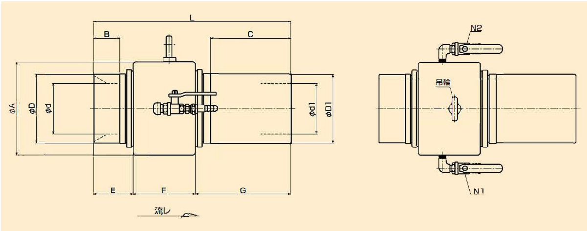
■ M472K-100B～M472K-150B寸法表（標準品）
