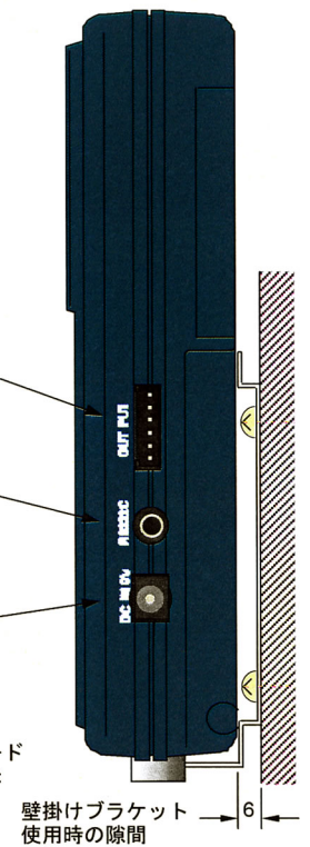
右側面
