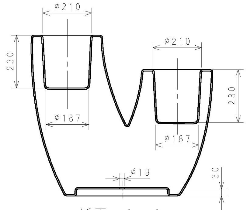
断面 A-A
