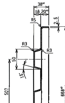
A-A' 断面詳細図 S=1:3
